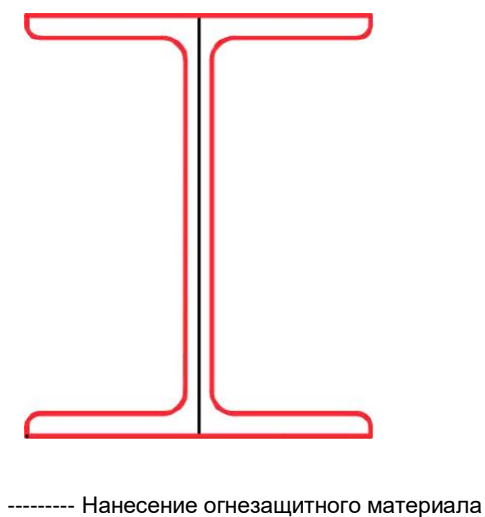
Рисунок Д.2 — Схема двутавровой балки с нанесенным огнезащитным материалом
